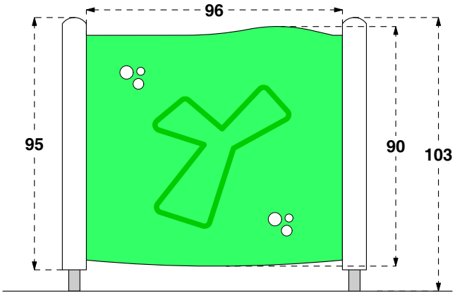
art. 200933 kit parapetto 96x90 young
