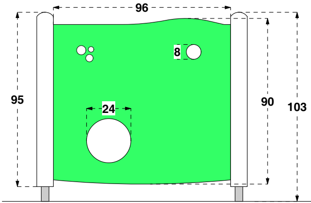
art. 200946 kit parapetto con 2 fori young
