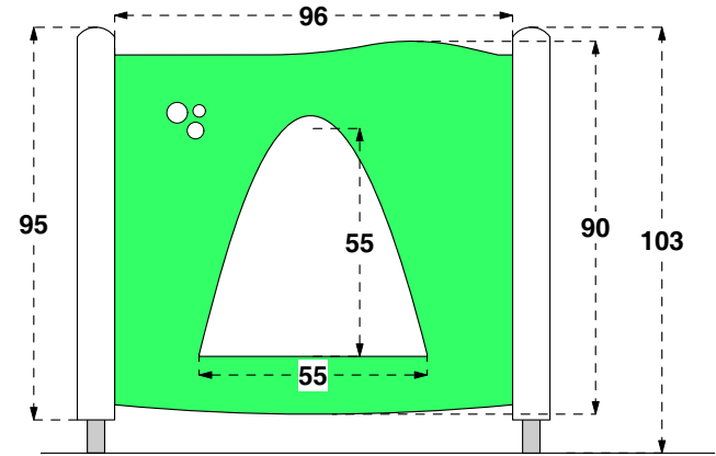
art. 200945 kit parapetto con cuspidate young
