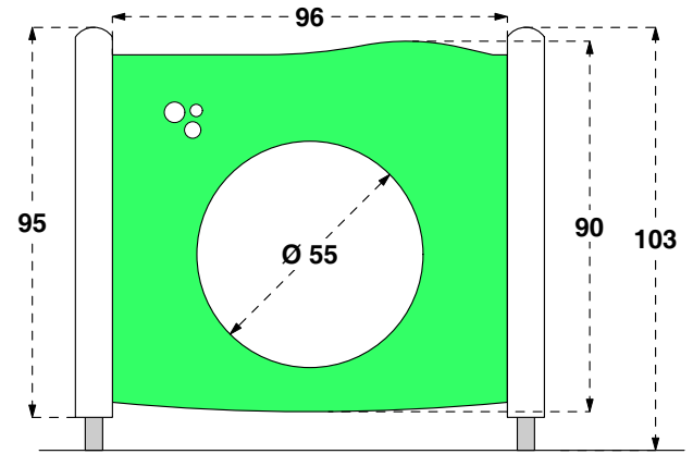
art. 200947 kit parapetto con foro grande young
